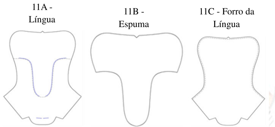
Figura 11 – Peças da Lingueta
