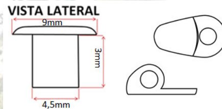
Figura 15 – Ilhós Redondo Latão 51 e Ilhós Gancho Zamac
